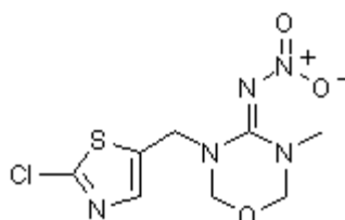
31 CGA 293343 Novartis
