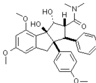
80 rocaglamide
