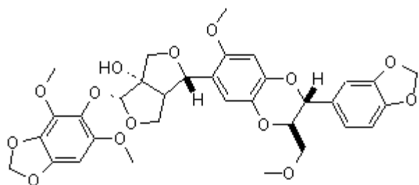
79 haedoxan A
