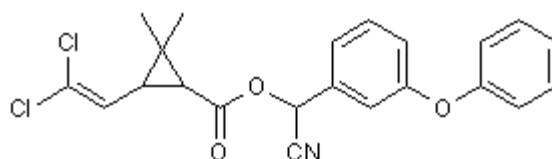
14 cypermethrin Rothamstead
