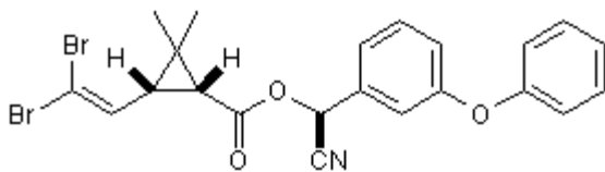
15 deltamethrin Rothamstead
