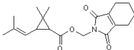
5 tetramethrin Sumitomo
