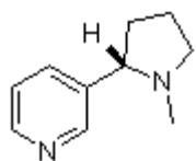
23 nicotine
