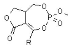
80 rocaglamide
