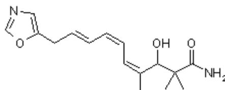
133 phthoxazolin A
