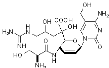
101 mildiomyacin
