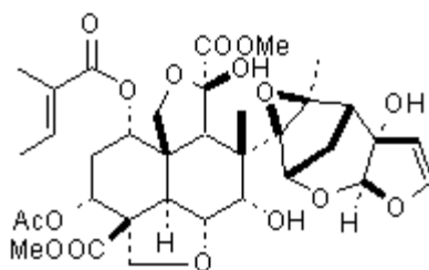
59 Azadirachtin
