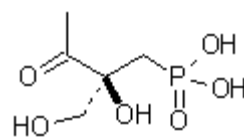
130 phosphinothrixin
