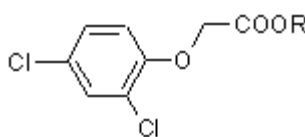
115 2,4-D
