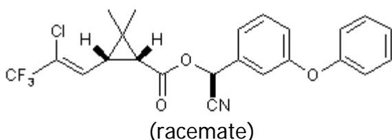
17 [lambda]-cyhalothrin ICI (now Zeneca)
