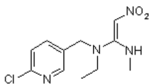
26 nitenpyram Takeda
