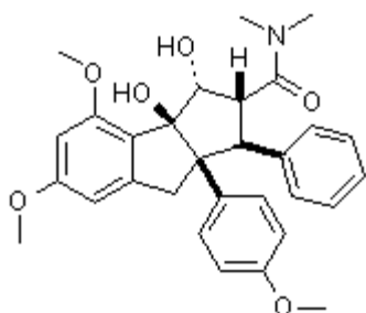
80 rocaglamide
