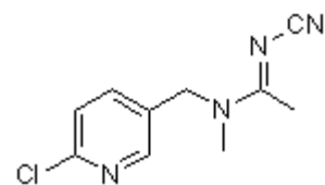
27 acetamiprid Nippon Soda
