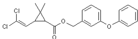
13 permethrin Rothamstead
