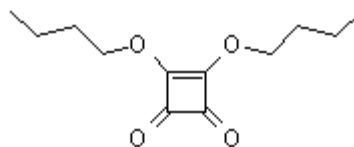
135 CGA 49445
