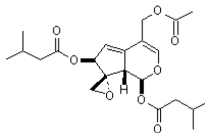
113 valtrate
