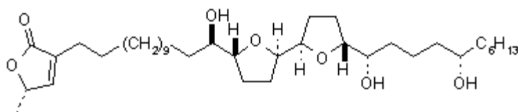
78 annonin I
