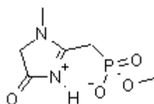
84 ulosantoin
