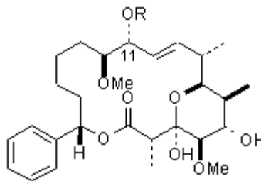
102 R = CH 3 : soraphen A
