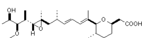
132 herboxidiene
