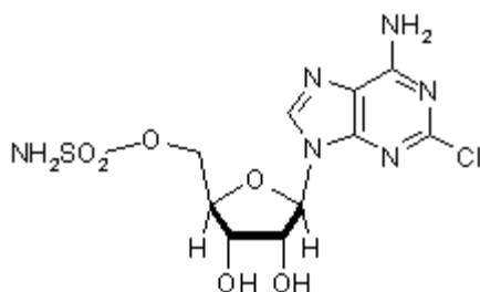
126 AT-265
