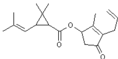
3 allethrin USDA
